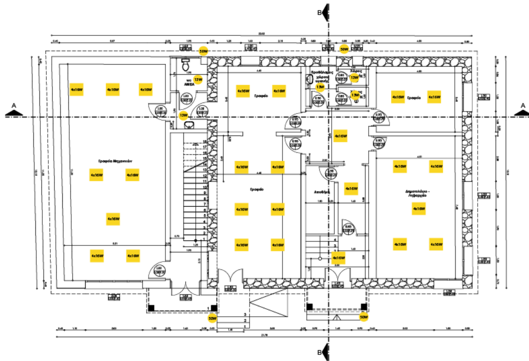
Εικόνα 28 Τα φώτα του ισογείου
