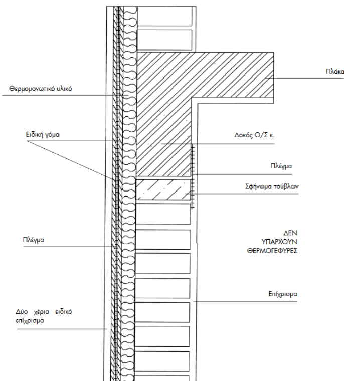
Εικόνα 37 Εξωτερική θερμομόνωση τοίχου με μονωτικό υλικό
