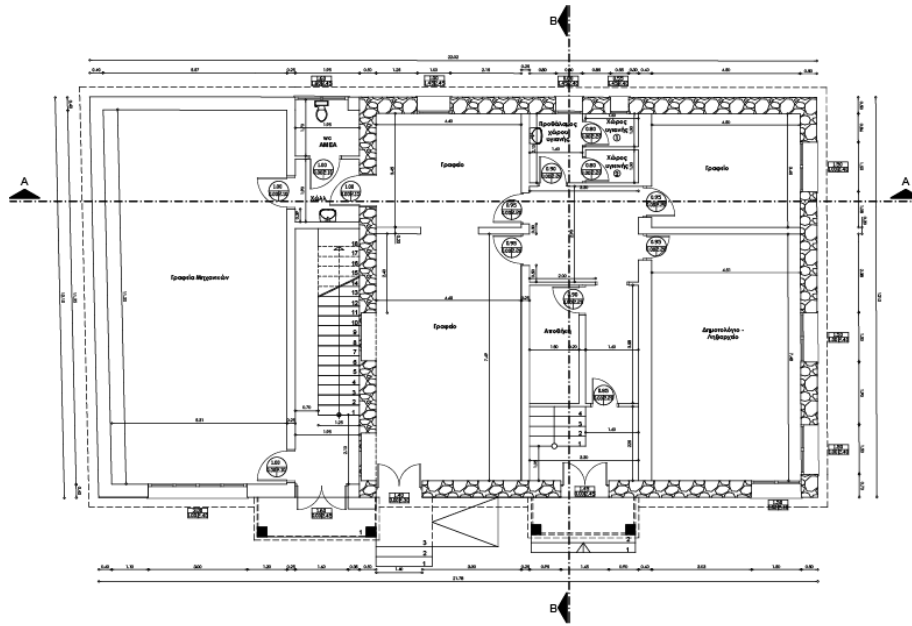
Εικόνα 10 Κάτοψη Ισογείου
