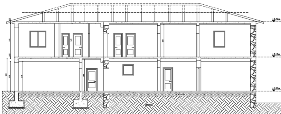
Εικόνα 12 Τομή α-α'
