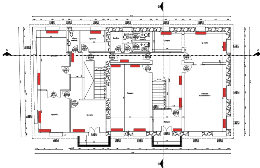
Εικόνα 41 Θέση των calorifέρ στον όροφο
