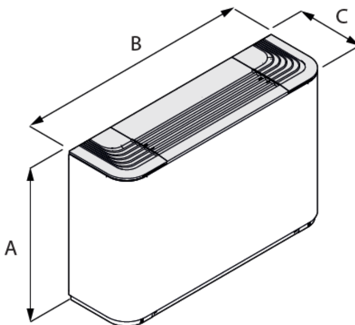
Εικόνα 49 Διαστάσεις του fan-coil
