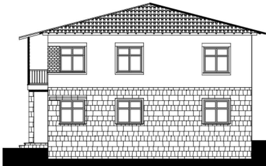
Εικόνα 15 Ανατολική όψη
