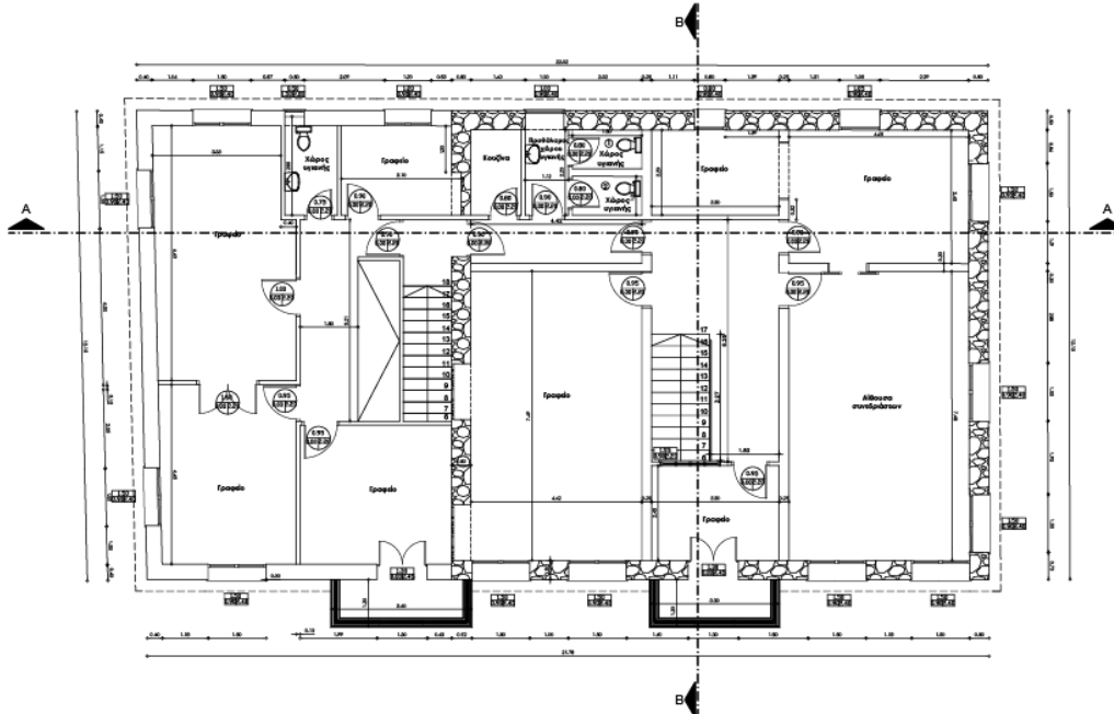
Εικόνα 11 Κάτοψη ορόφου
