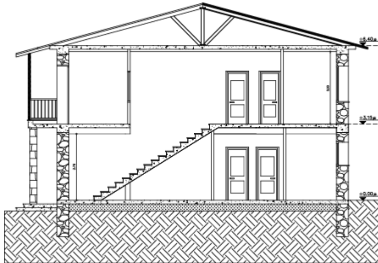
Εικόνα 13 Τομή β-β'
