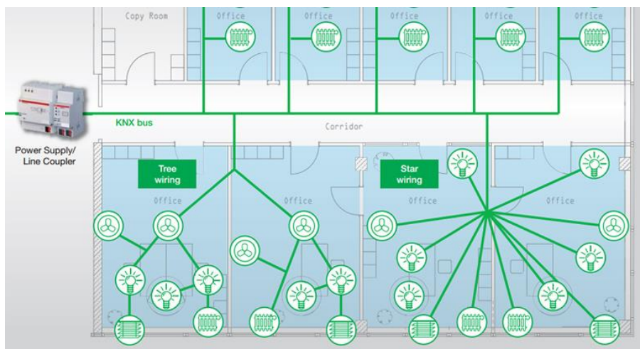
Εικόνα 52 Σύστημα KNX
